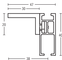
Supporto a soffitto 0-8 mm Articolo n. 11588
