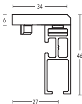
Supporto a soffitto 6 mm Articolo n. 11590-1
