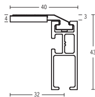
Supporto a soffitto 3 mm Articolo n. 11597
