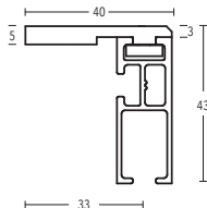
Supporto a soffitto 3 mm Articolo n. 11592
