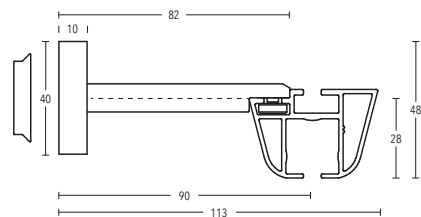
Wandträger Art.-Nr. 11260-90
