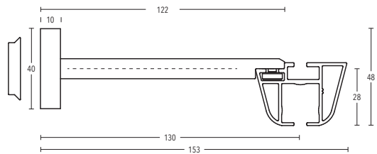
Wandträger Art.-Nr. 11260-130
