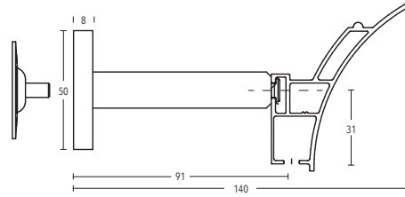
Wandträger Art.-Nr. 11478
