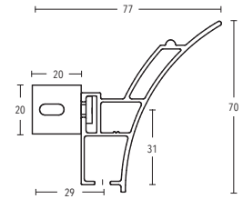
Wandlager mit Winkeldeckenträger Art.-Nr. 11591-00
