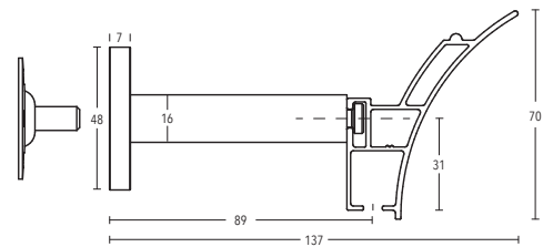
Wandträger Art.-Nr. 11873-80
