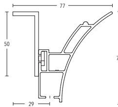
Winkel-Deckenträger 3 mm Art.-Nr. 11591-00
