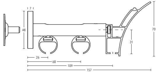
Multi-Wandträger 100 mm Art.-Nr. 11373-100
