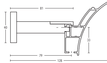
Klick-Wandträger Art.-Nr. 11808-80
