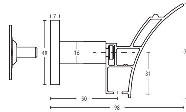
Wandträger Art.-Nr. 11873-50
