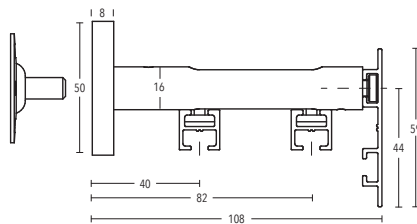
Wandträger 100 mm Art.-Nr. 11173-100
