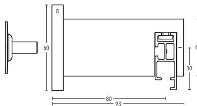
Wandträger Art.-Nr. 11570-80
