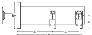
Wandträger Art.-Nr. 11570-2 + 11570-2-190
