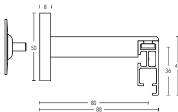
Wandträger Art.-Nr. 11460
