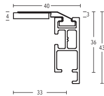
Deckenträger 3 mm Art.-Nr. 11597
