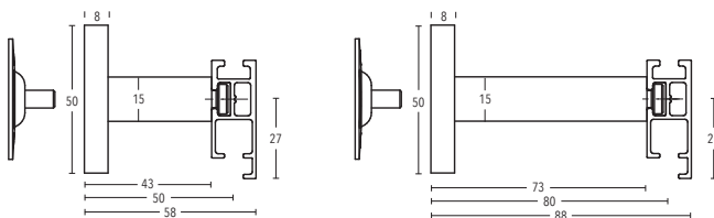
Wandträger Art.-Nr. 11473-50 + 11473-80
