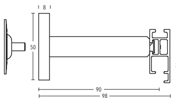
Wandträger Art.-Nr. 11478
