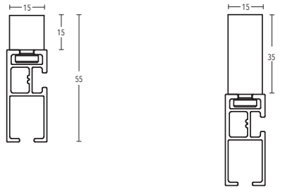
Wandträger Art.-Nr. 11473-50 + 11473-80
