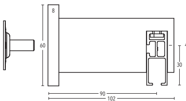
Wandträger Art.-Nr. 21570-90
