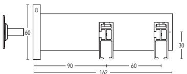
Wandträger Art.-Nr. 21570-150 + 21570-190
