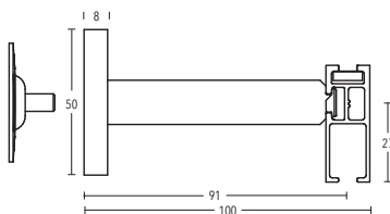
Wandträger Art.-Nr. 11478
